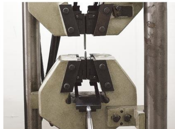
▲ 原材料拉力实验 Raw Material Tension Test
