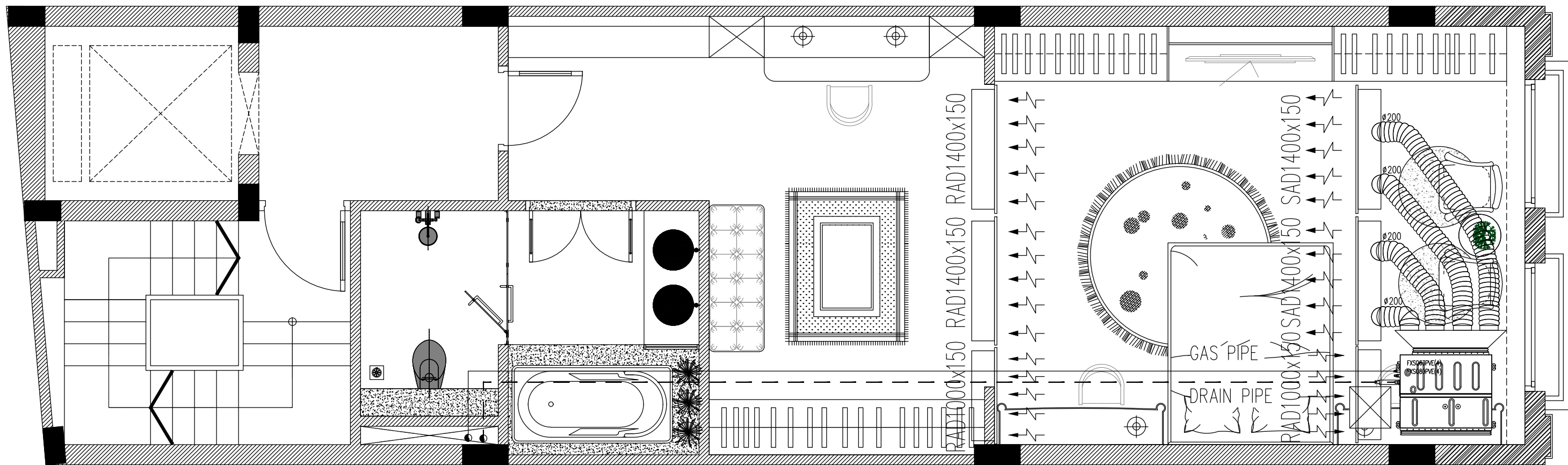
01 MẶT BẰNG TẦNG 5 A 3 TỶ LỆ 1/25
